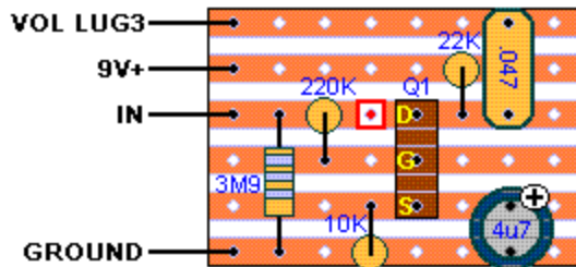
6 STRIPS X 8 HOLES Q1: NTE458
