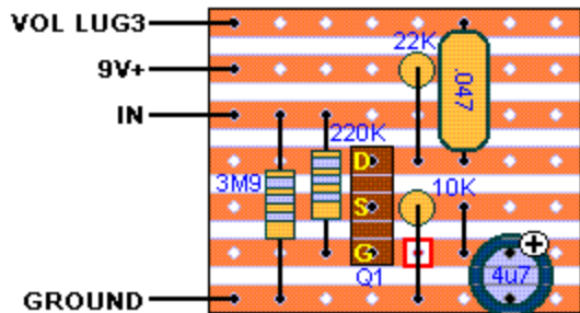
7 STRIPS X 8 HOLES Q1: J201 OR MPF102
