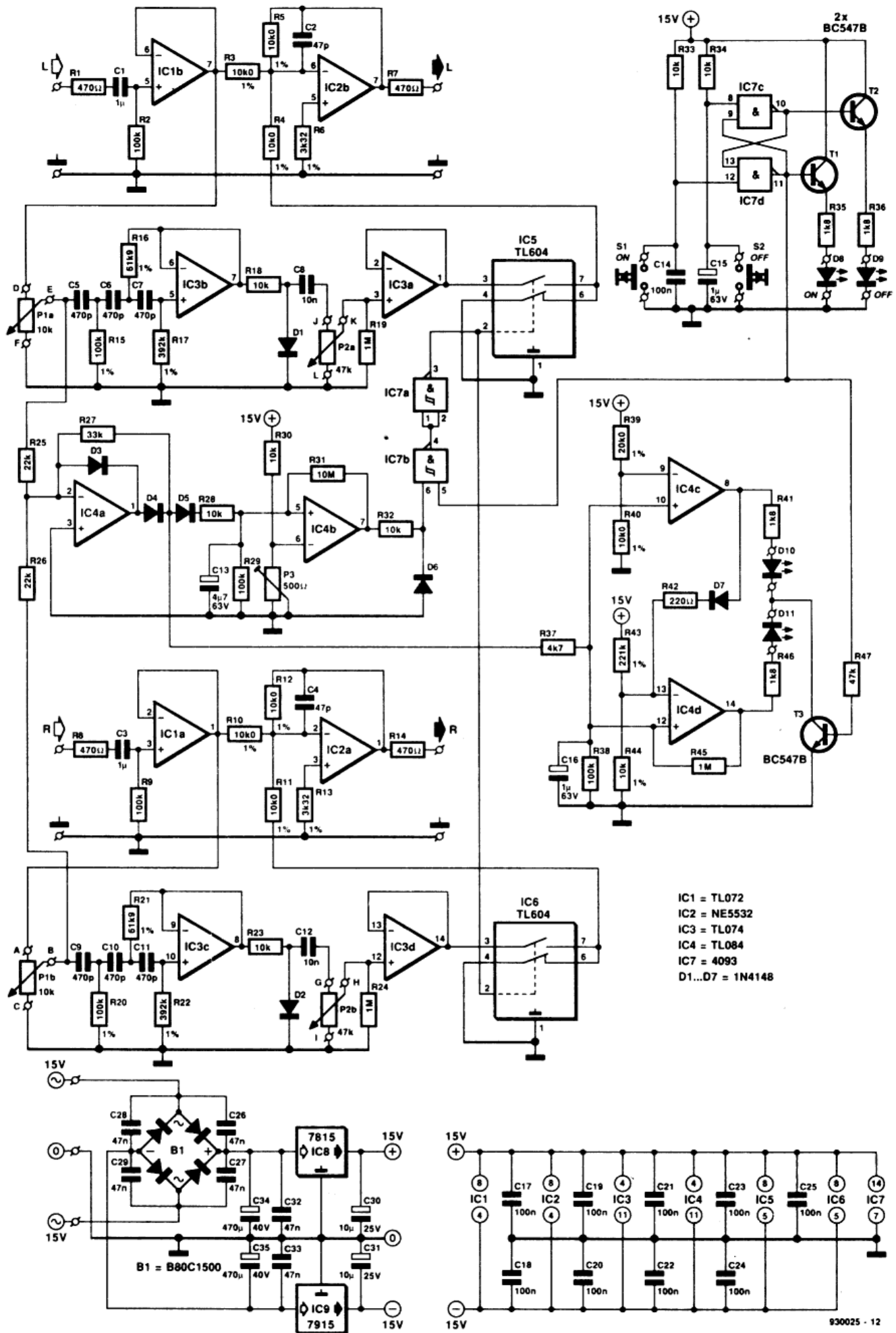
2. Schemat elektryczny wzmacniacza harmonicznych
