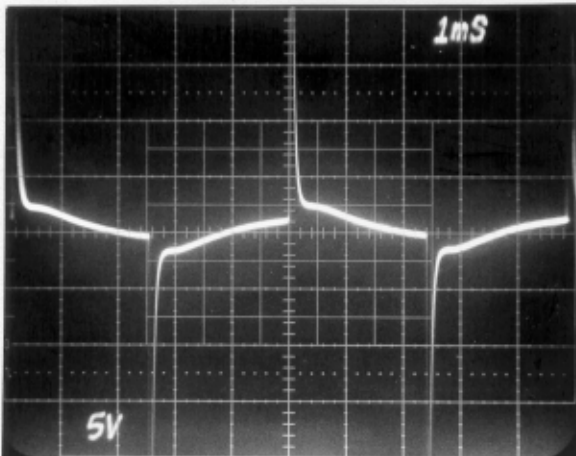
Fig. 12. Hi-Boost in.
